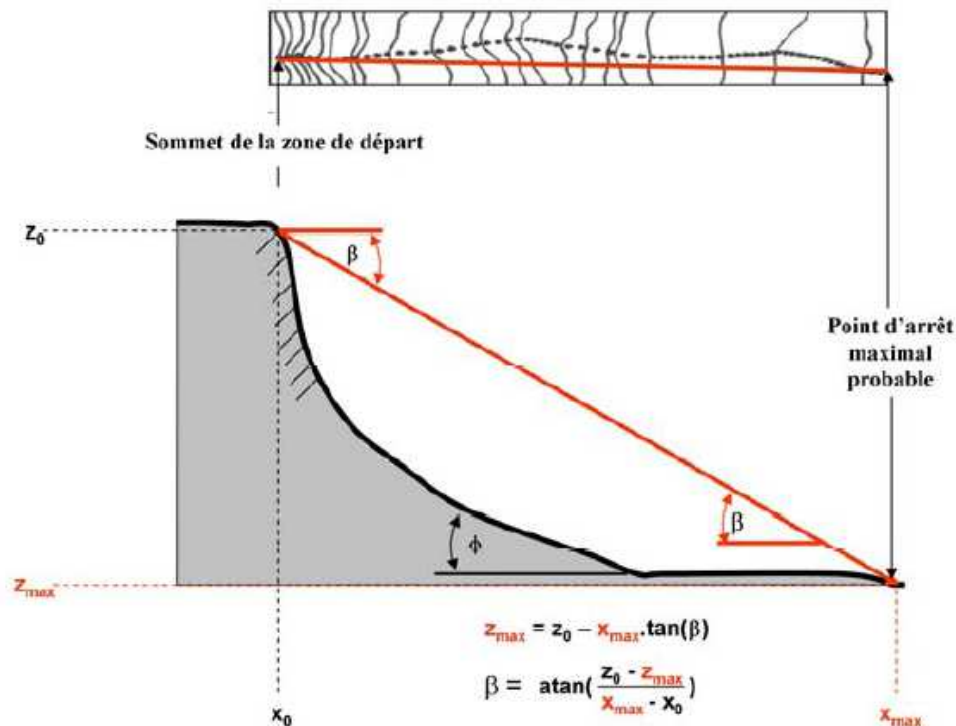
Illustration 5 - Schéma du principe d'évaluation de la ligne d'énergie
